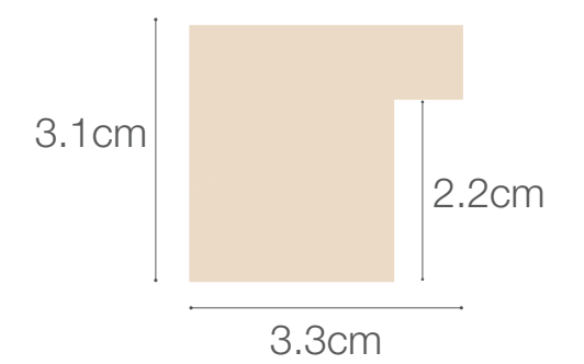
Profile: 6555#
